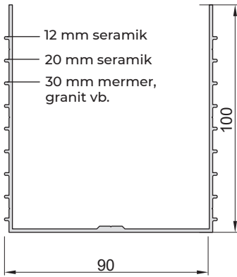
Smart Base 28 Kanal Profili
